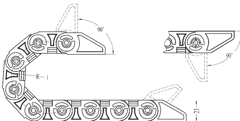
ОСНОВНЫЕ РАЗМЕРЫ КОНЦЕВЫХ ЭЛЕМЕНТОВ
